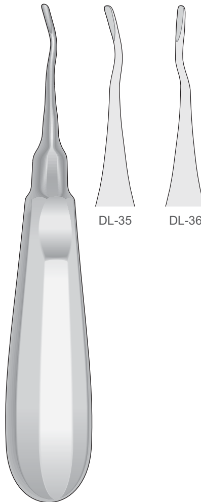
APEXO DL-35/DL-36 160 mm
